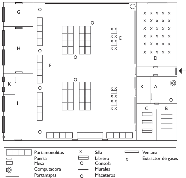
Figura 1. Diseño de las instalaciones de un Centro de Información Ecológica, Ambiental, Agropecuaria y Forestal. A) oficina; B) mapoteca, C) minibiblioteca, D) sala de conferencias, E) sala de consultas, F) sala de exposiciones, G) bodega H) cuarto de preparación de monolitos de suelos, I) laboratorio, J) pasillo lateral y K) sanitario.
